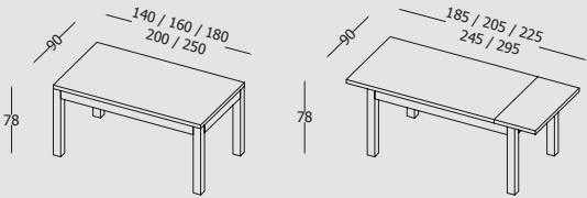
Tavolo allungabile con gambe in massello di frassino e piano impiallacciato sp. 4 cm. Extendable table with solid ash legs and 4 cm thick veneered top.
