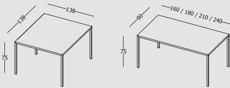
Tavolo fisso interamente in metallo verniciato opaco goffrato. Gambe in metallo con sezione 3x3 cm. Fixed table made entirely of embossed matte painted metal. Metal legs with 3x3 cm section.
