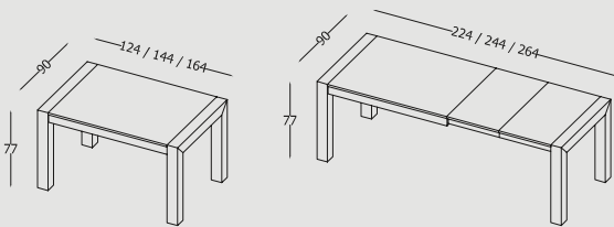
Tavolo allungabile impiallacciato con piano sp. 2 cm e gambe in legno massello sezione 10x9 cm. Veneered extendable table with 2 cm thick top and solid wood legs with 10x9 cm section.
