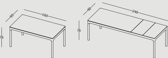
Tavolo allungabile con gambe in massello di frassino e piano impiallacciato sp. 1 cm. Extendable table with solid ash legs and 1 cm thick veneered top.
