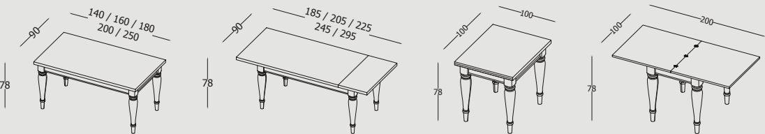
Tavolo allungabile con struttura impiallacciata e gambe in massello e con piano impiallacciato sp. 4 cm. Extendable table with veneered structure, solid wood legs, and 4 cm thick veneered top.
