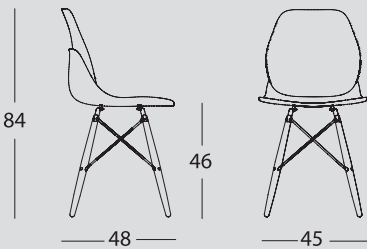
Sedia con gambe in faggio, struttura in metallo verniciato nero e seduta in polipropilene. Chair with beech legs, black painted metal structure and polypropylene seat.
