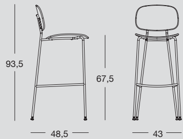
Sgabello con struttura in acciaio verniciato o cromato, seduta e schienale in poliropilene. Stool with painted steel or chrome-plated structure, and polypropylene seat and back.
