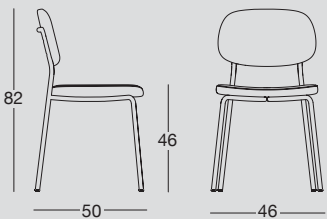
Sedia con struttura in metallo verniciato e seduta imbottita e rivestita in velluto antimacchia. Chair with painted metal structure and padded seat upholstered in stainproof velvet.
