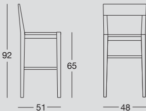
Sgabello con struttura in legno e seduta impagliata o legno. Stool with wood structure and rush or wood seat.
