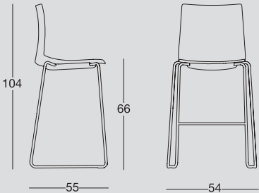
Sgabello con struttura in metallo verniciato e seduta in tecnopolimero. Stool with painted metal structure and technopolymer seat.
