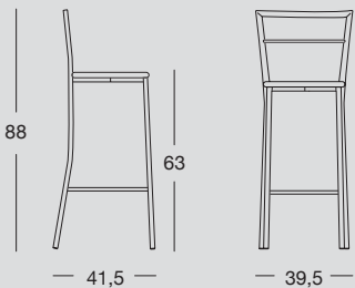
Sgabello con struttura tubolare in metallo, seduta in multistrato laccato opaco. Stool with tubular metal structure and matte lacquered plywood seat.
