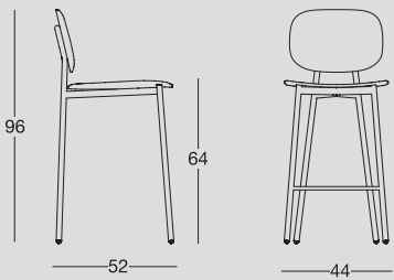
Sgabello con struttura in metallo verniciato, seduta in polipropilene rinforzato fibra vetro. Stool with painted metal structure, polypropylene seat reinforced with fibreglass.
