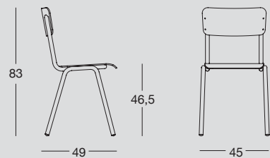
Sedia con struttura in metallo grezzo verniciato trasparente o brunito con seduta e schienale in multistrato. Chair with transparent painted or burnished raw metal structure, with plywood seat and back.
