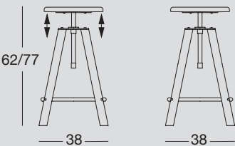
Sgabello con struttura e seduta in legno con poggiapiedi e dettagli in metallo verniciato lucido grigio scuro. Stool with wood structure and seat with dark grey glossy painted metal details and footrest.
