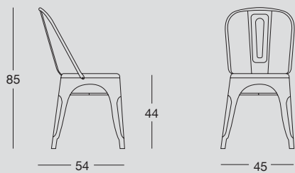
Sedia in metallo verniciato naturale, anticato o brunito. Chair in antique or burnished natural painted metal.
