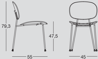
Sedia con struttura in acciaio verniciato o cromato, seduta e schienale in multistrato di rovere. Chair with painted steel or chrome-plated structure, and oak plywood seat and back.
