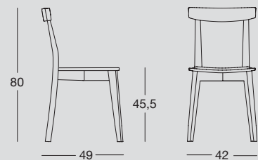
Sedia con struttura in legno massello di faggio laccato e seduta in multistrato laccato. Chair with lacquered solid beech wood structure and lacquered plywood seat.
