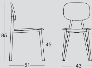
Sedia con struttura in acciaio, giunto in alluminio, seduta e schienale in polipropilene. Chair with steel structure, aluminium joint, polypropylene seat and back.
