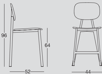
Sgabello con struttura in acciaio e giunto in alluminio, seduta e schienale in polipropilene. Stool with steel structure, aluminium joint, polypropylene seat and back.
