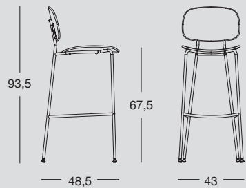
Sgabello con struttura in acciaio verniciato o cromato, seduta e schienale in multistrato di rovere. Stool with painted steel or chrome-plated structure, and oak plywood seat and back.
