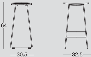
Sgabello con struttura in acciaio verniciato o cromato e seduta in frassino. Stool with painted steel or chrome-plated structure, and ash seat.
