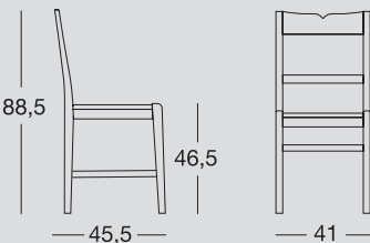
Sedia con struttura in legno e seduta impagliata o in legno. Chair with wood structure and rush wood seat.
