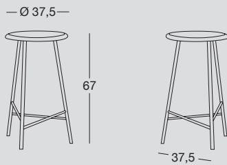
Sgabello con struttura in metallo verniciato e seduta in legno. Stool with painted metal structure and wood seat.
