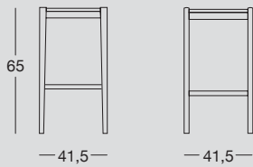
Sgabello con struttura in legno e seduta impagliata o legno. Stool with wood structure and rush or wood seat.
