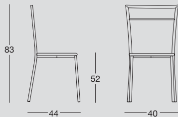
Sedia con struttura realizzata in tubolare metallico e seduta in multistrato laccato opaco. Chair with tubular metal structure and matte lacquered plywood seat.
