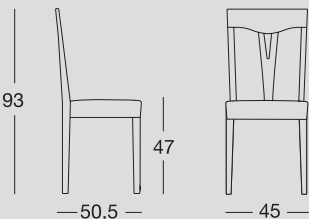
Sedia con struttura in legno con seduta impagliata o legno. Chair with wood structure and rush or wood seat.
