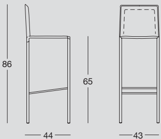
Sgabello con struttura in metallo, imbottito e completamente rivestito in ecopelle e poggia piedi in metallo cromato. Stool with metal structure, padded and entirely upholstered in eco-leather, with chrome-plated metal footrest.
