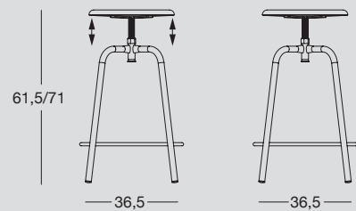
Sgabello con struttura in metallo verniciato e seduta in legno. Stool with painted metal structure and wood seat.
